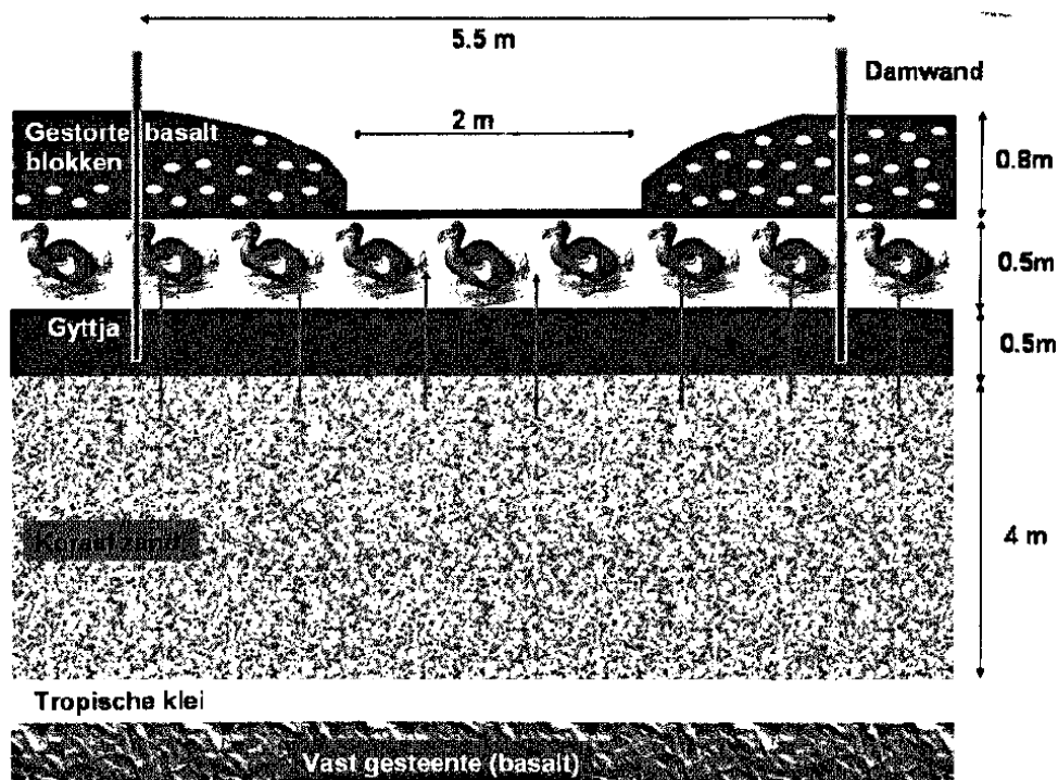
Figuur 1. Geologisch profiel van opgraving A in Mare aux Songes en een schematische weergave van de Dodopolder (de Louw en Rijdsdijk, 2007)
